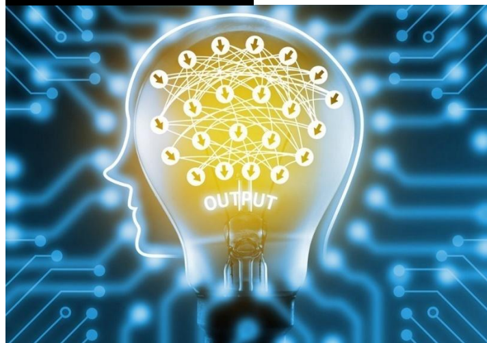
類神經網絡
